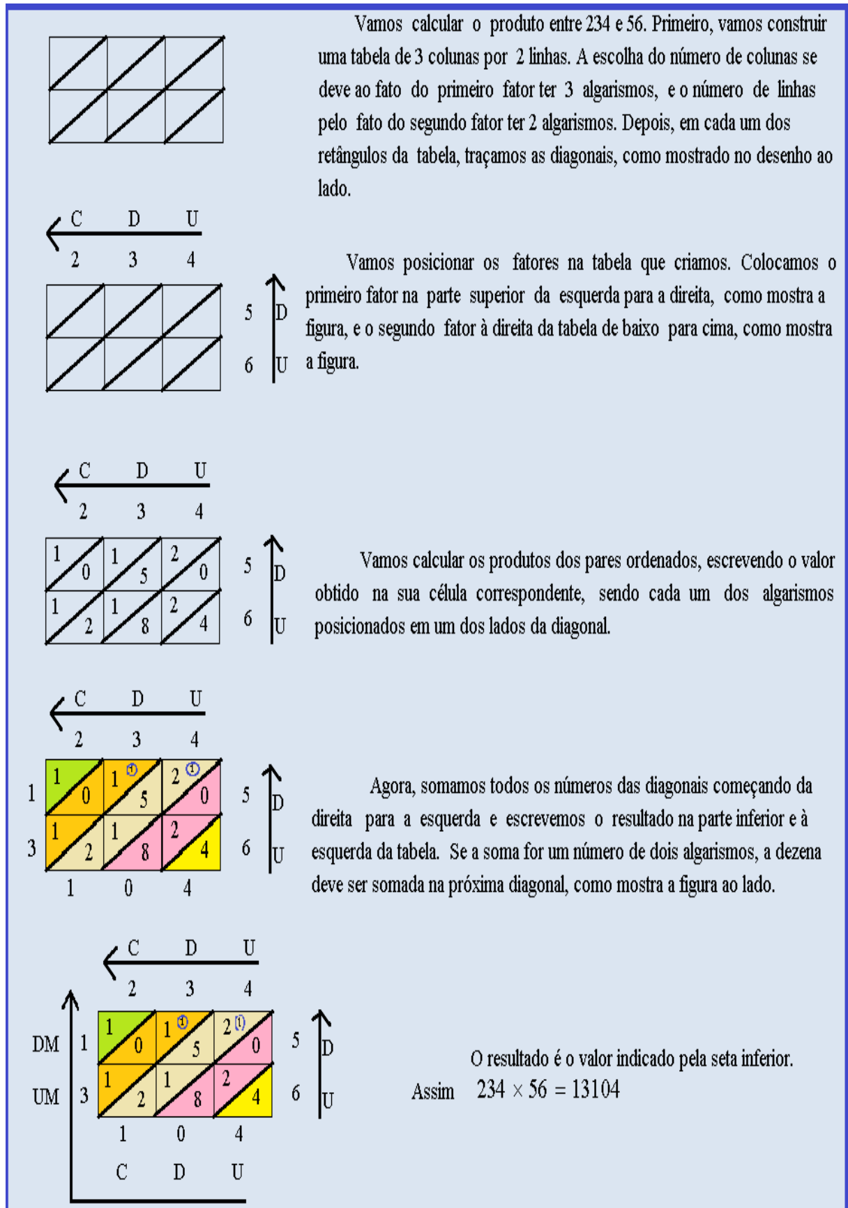
Figura 114: Algoritmo da multiplicação usando tabela
