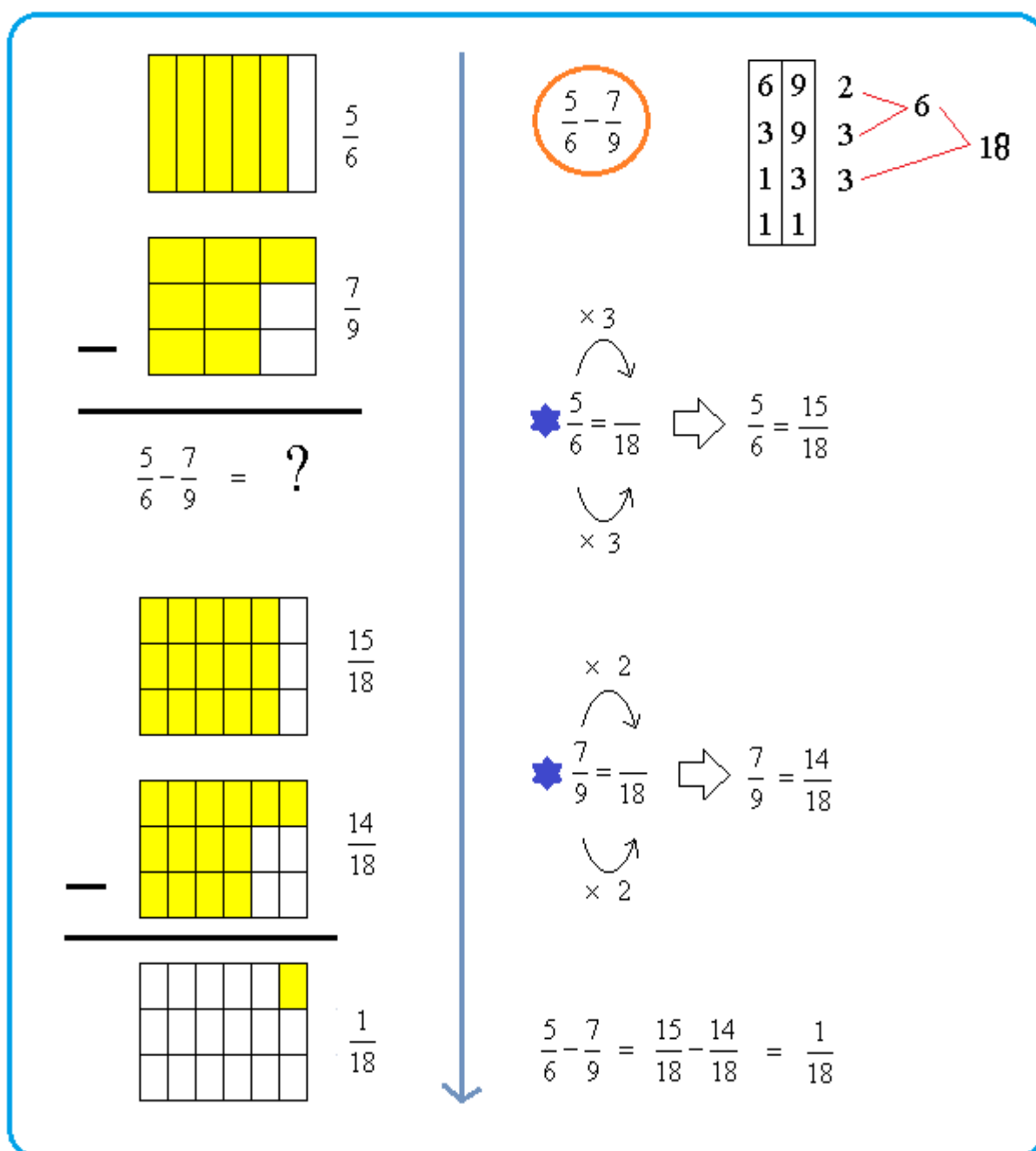
Figura 167: Subtração com frações
