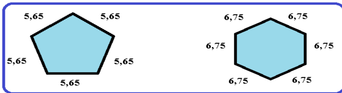
Figura 183: Pentágono e hexágono
