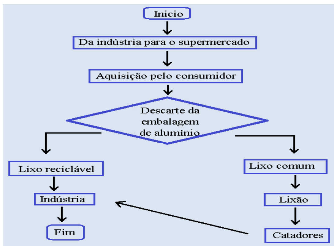
Figura 220: Fluxograma 1
